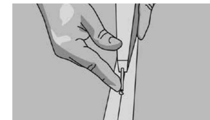
Рис. 43. Всегда работайте двумя руками! Одной рукой держите тубик, указательный палец второй руки положите на сопло. Вдавите иглу глубоко в шов так, чтобы холодная сварка попала в образовавшееся отверстие.
